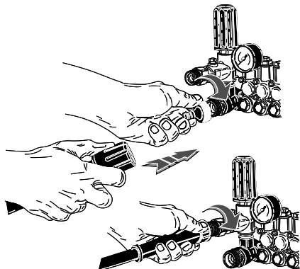
Tilslutning til vandforsyningen.
